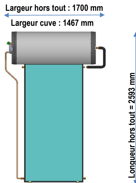
Vue en plan (en vraie grandeur)
