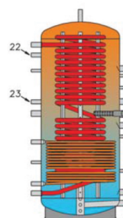
TSPU : avec 1 échangeur à serpentin
